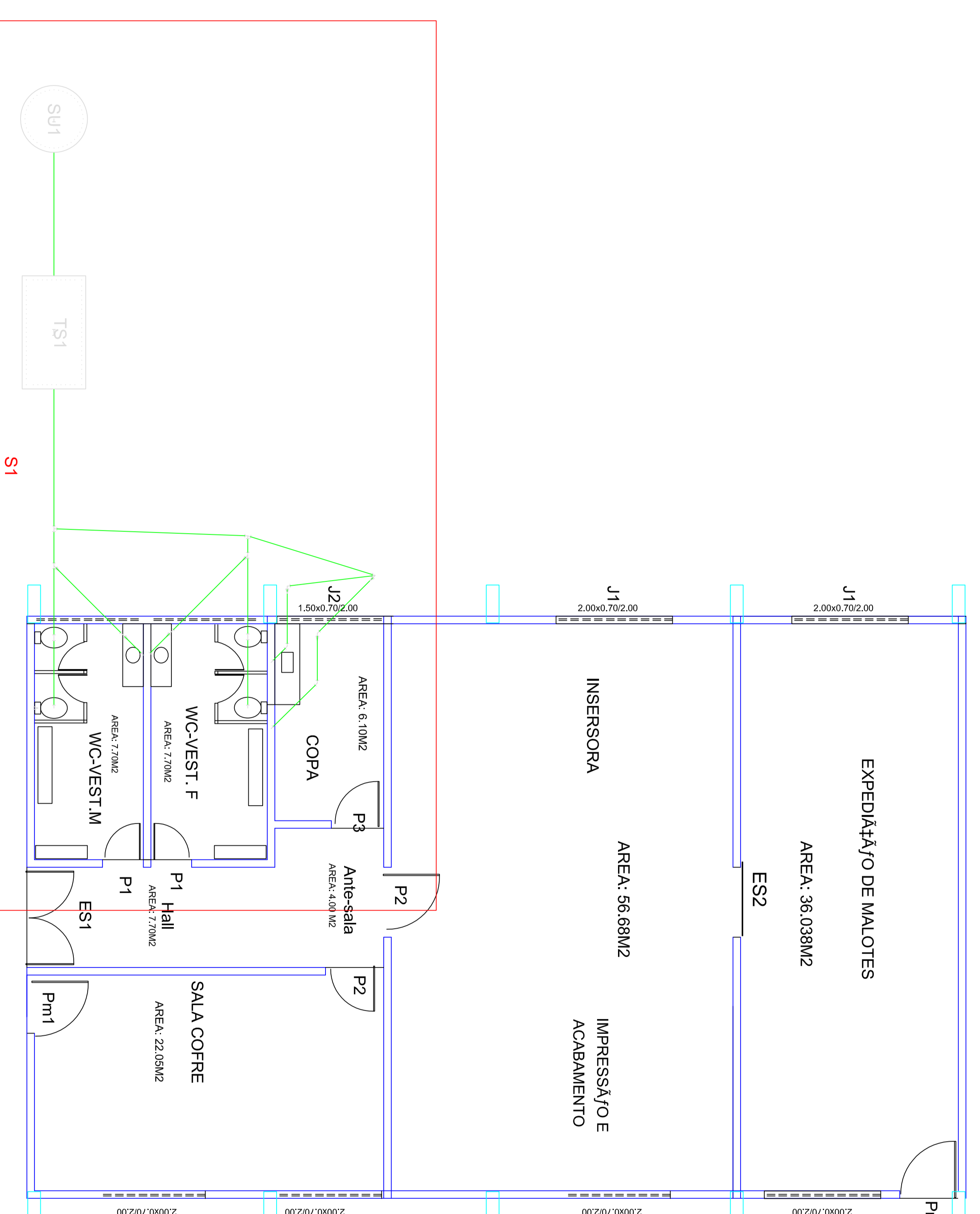
Planta baixa sanitário escala 1:50
