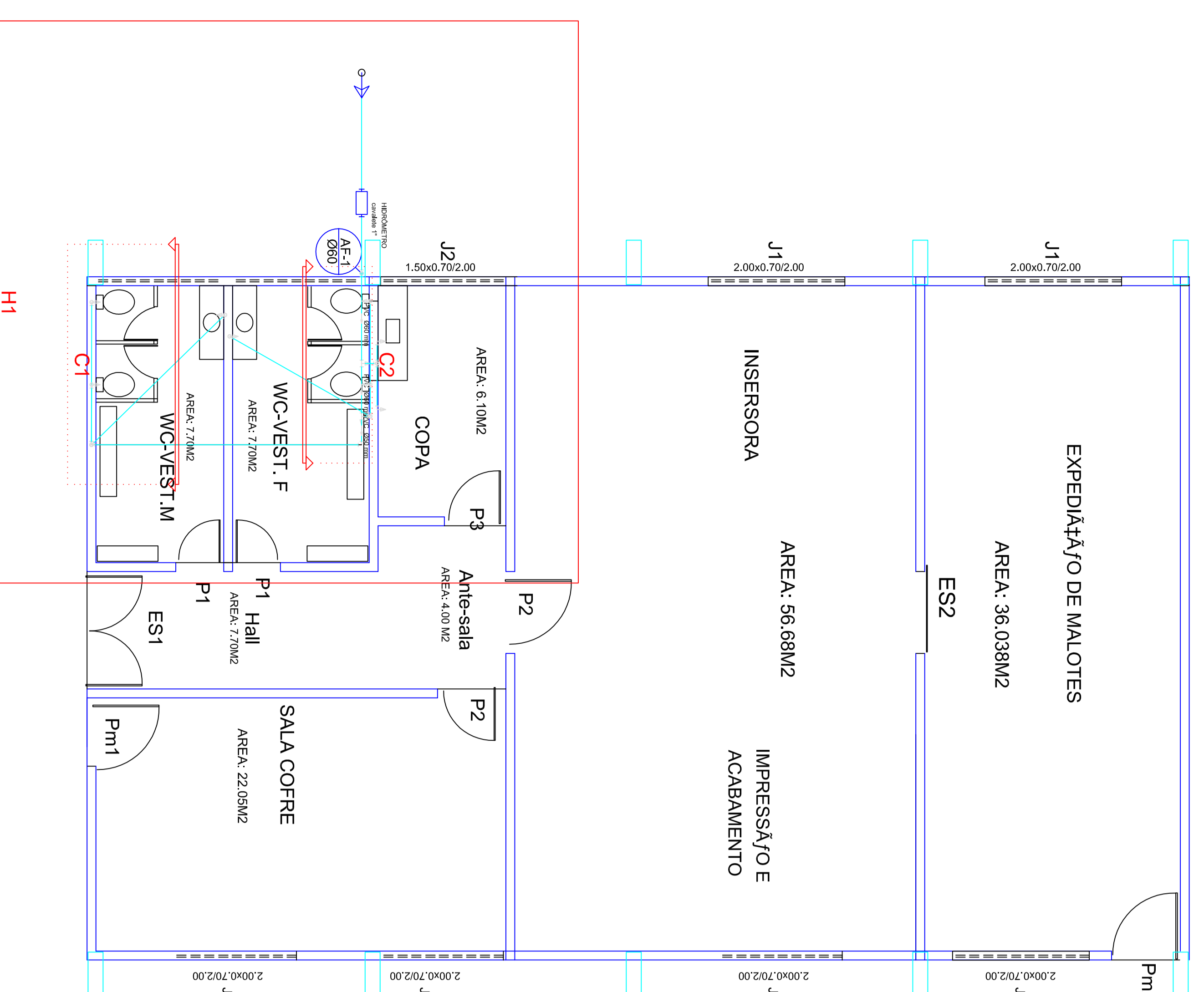
Planta baixa hidráulico escala 1:50
